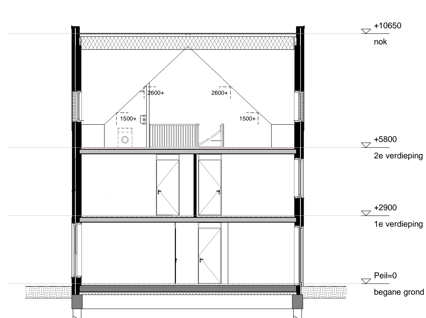
Doorsnede B9-A2
