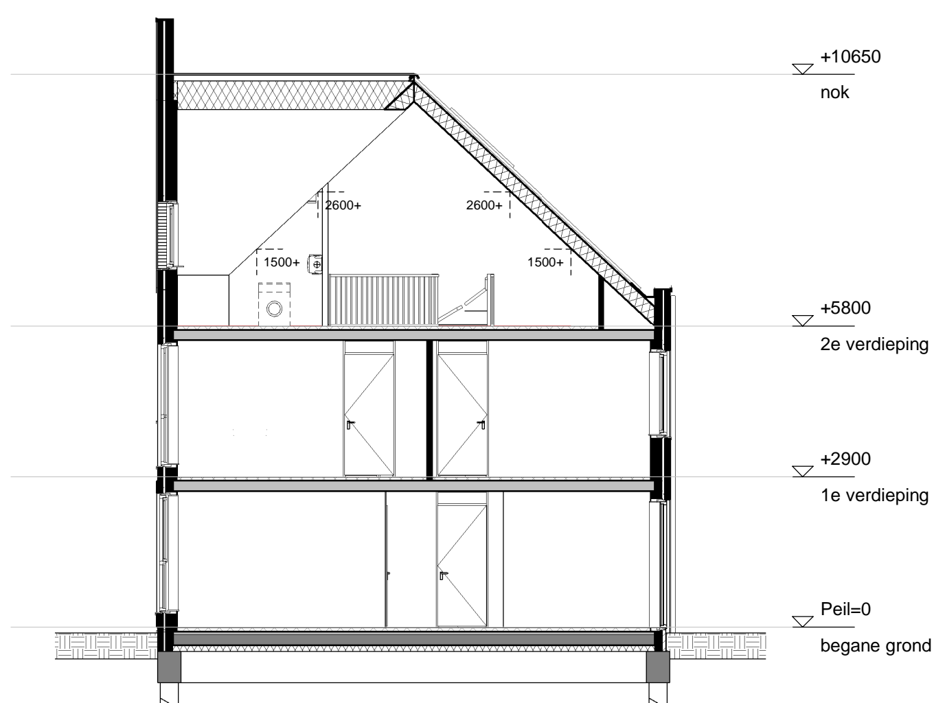
Doorsnede B9-A1
